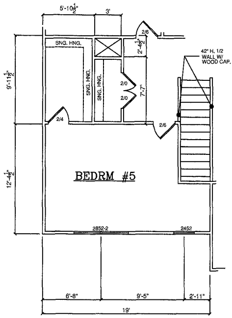
OPTIONAL BEDROOM #5 SCALE: 1/8"=1'-0"
